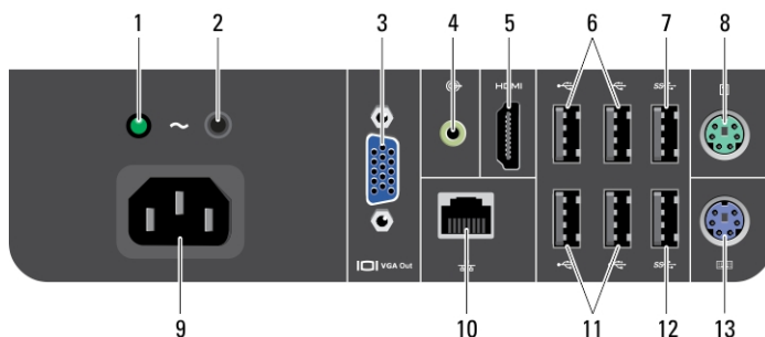
Рисунок 3. Вид задней панели
